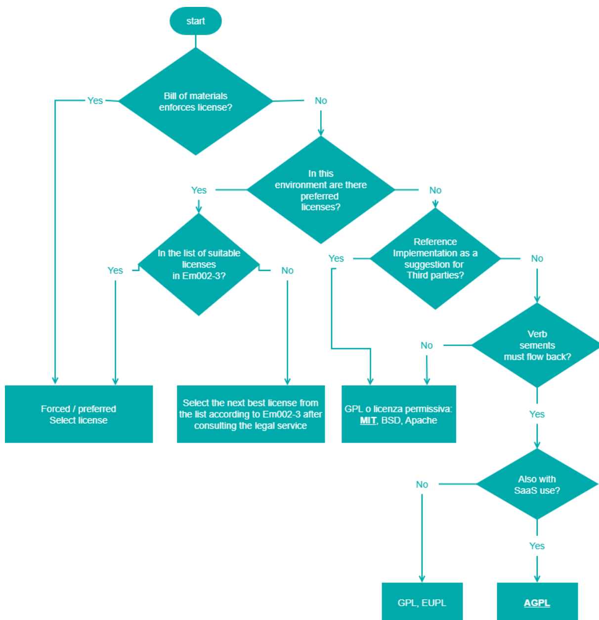
Figura 3: Albero decisionale ampliato per la scelta della licenza nell'Amministrazione federale (se non AGPL o MIT)
