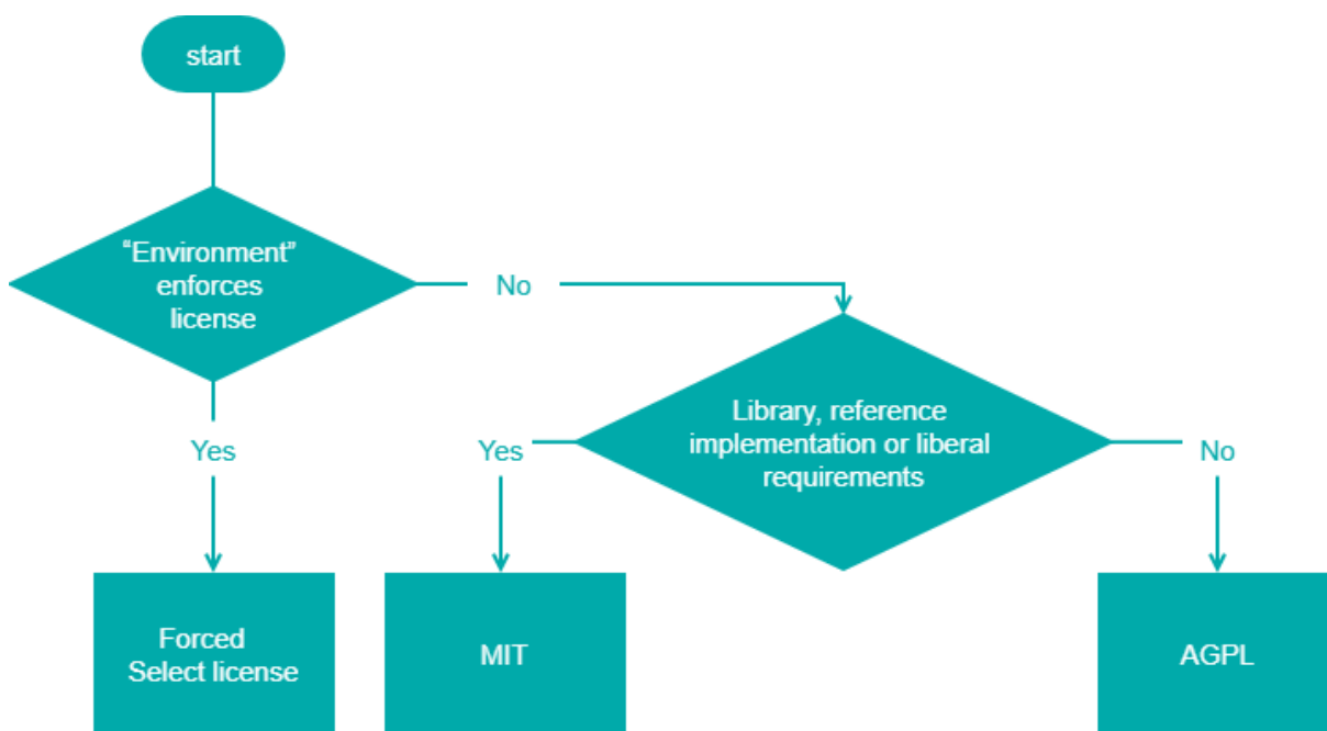
Figura 1: Ausilio decisionale semplificato per la scelta della licenza
