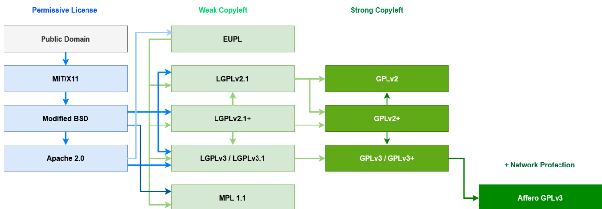
Figura 2: Compatibilità delle licenze open source (sulla base del grafico di David A. Wheeler, 2007 e di https://www.gnu.org/licenses/license-list.it.html )
