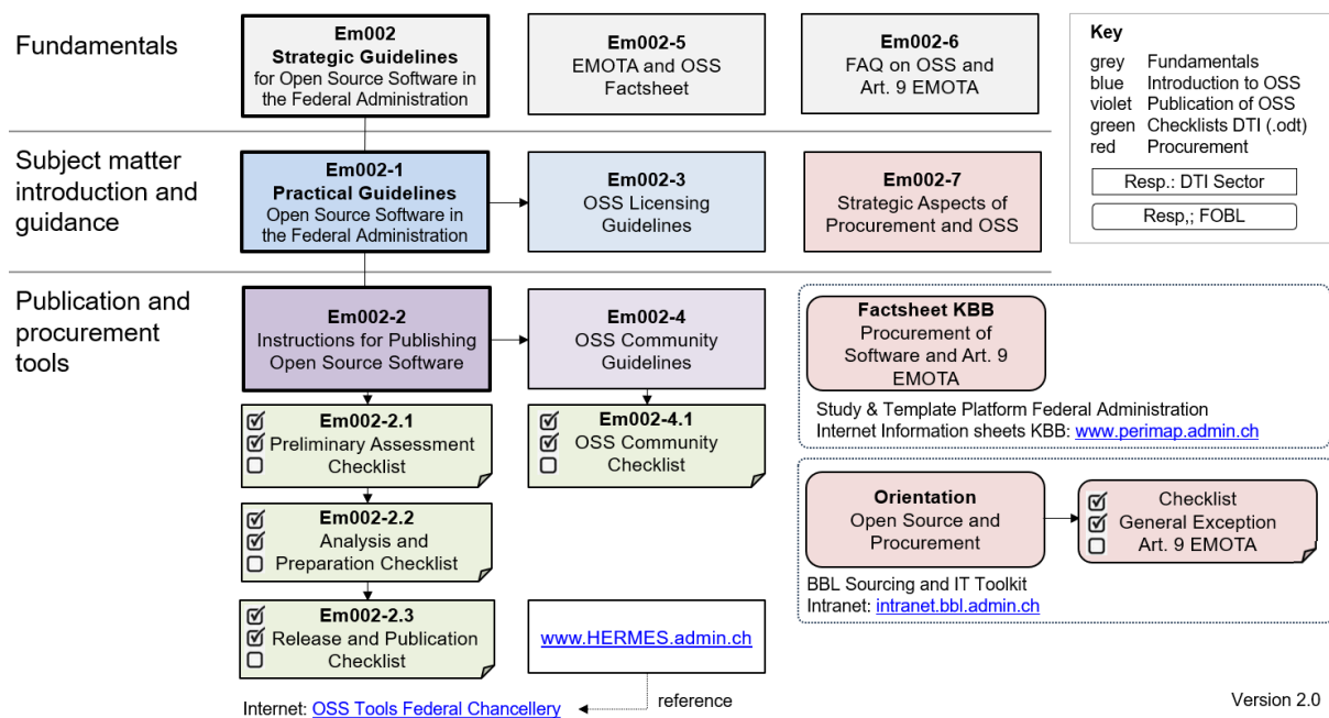
Illustraziun 1: Survista dals meds OSS
