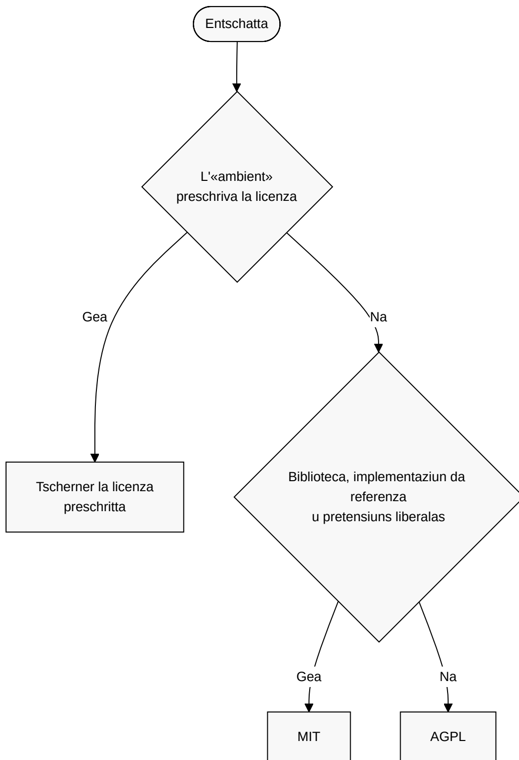
Illustraziun 1: Agid da decisiun simplifitgà per la tschernà da la licenza
