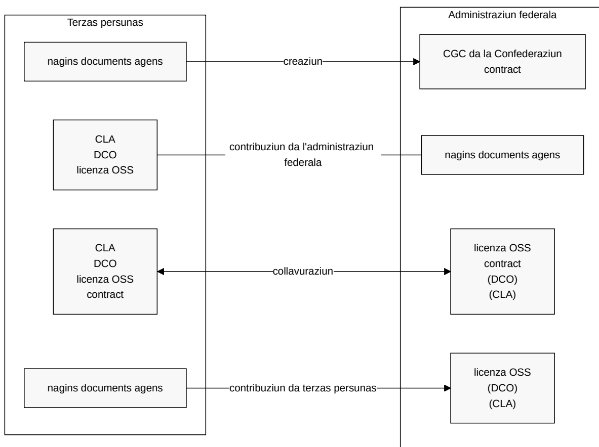
Illustraziun 4: Transferiment da code da funtauna e da dretgs en differentas constellaziuns
