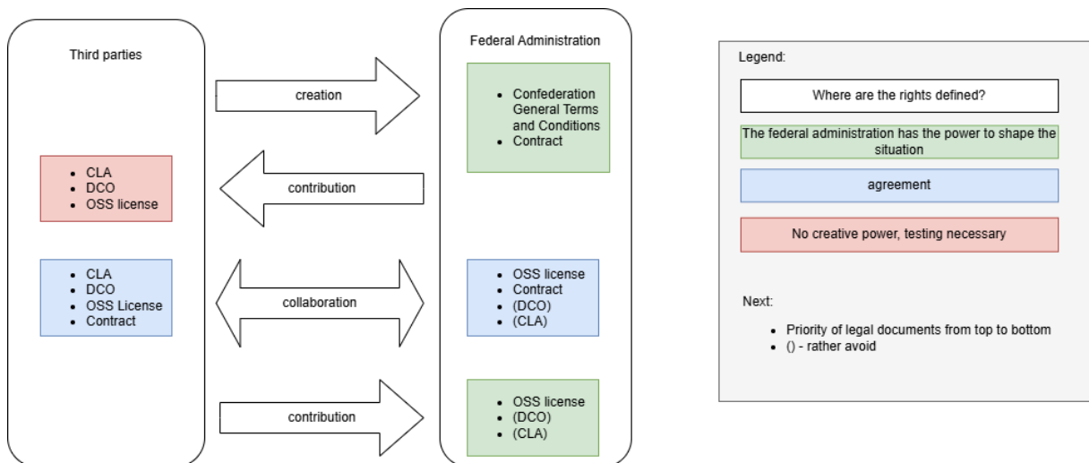
Figure 4 : Transfert du code source et des droits dans différentes constellations
