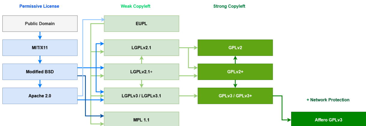
Figure 2 : Compatibilité des licences open source (d'après le schéma de David A. Wheeler, 2007 et https://www.gnu.org/licenses/license-list.fr.html )
